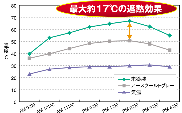
アスファルト面における温度比較 (弊社試験)
